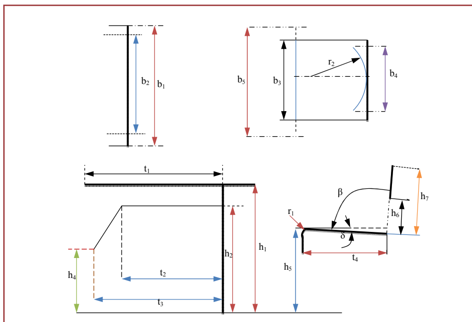
شکل ۶- ابعاد میز و صندلی در مدل BS5873
