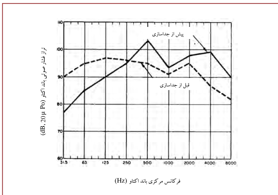
شکل ۳۰- ترازهای شبهه نقطه اوج ۴ ft از پایین دستگاه پرس پیش و بعد از جداسازی
